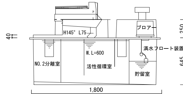
断面図 S=1:20 ウォータス本体 (下部装置)
